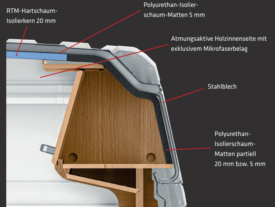
Malibu Van: aufwendige Karosserie-Isolationsmaßnahmen
