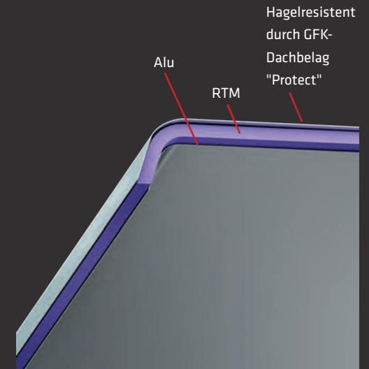
Malibu Van Hybrid-Aufstelldach mit klassenbestem Isolationskonzept in Sandwichbauweise und mit geringem Eigengewicht
